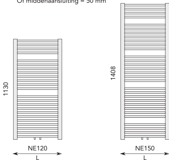
Vooraanzicht
