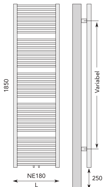
Zijaanzicht
